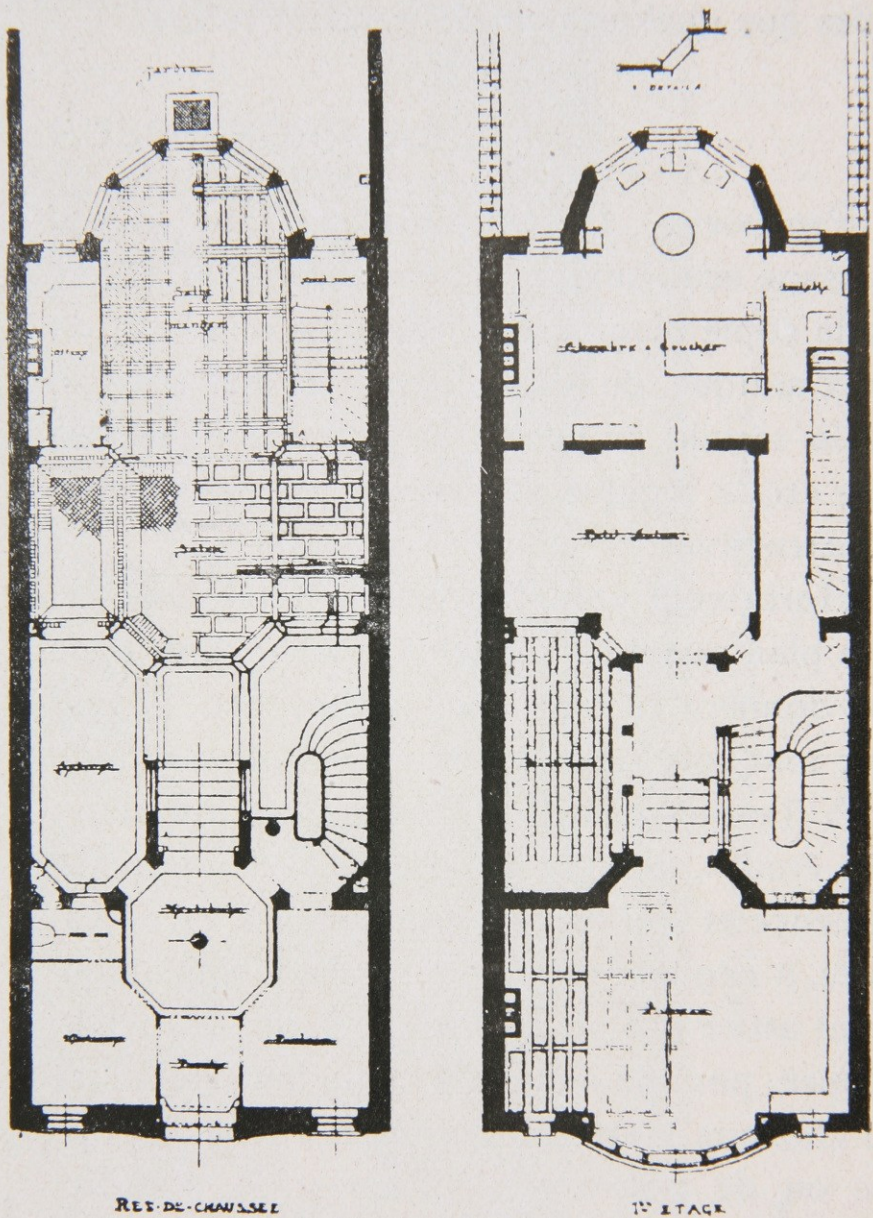
HOTEL DE M. TASSEL, RUE DE TURIN A BRUXELLES PLANS (V. HORTA, ARCH.)
